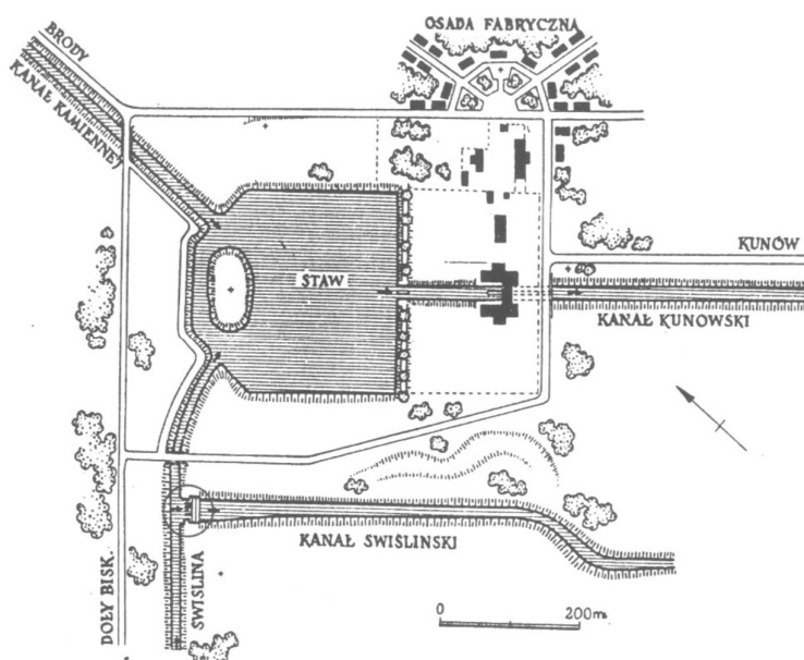
Rysunek 48. Walcownia w Nietulisku Dużym – układ przestrzenny
