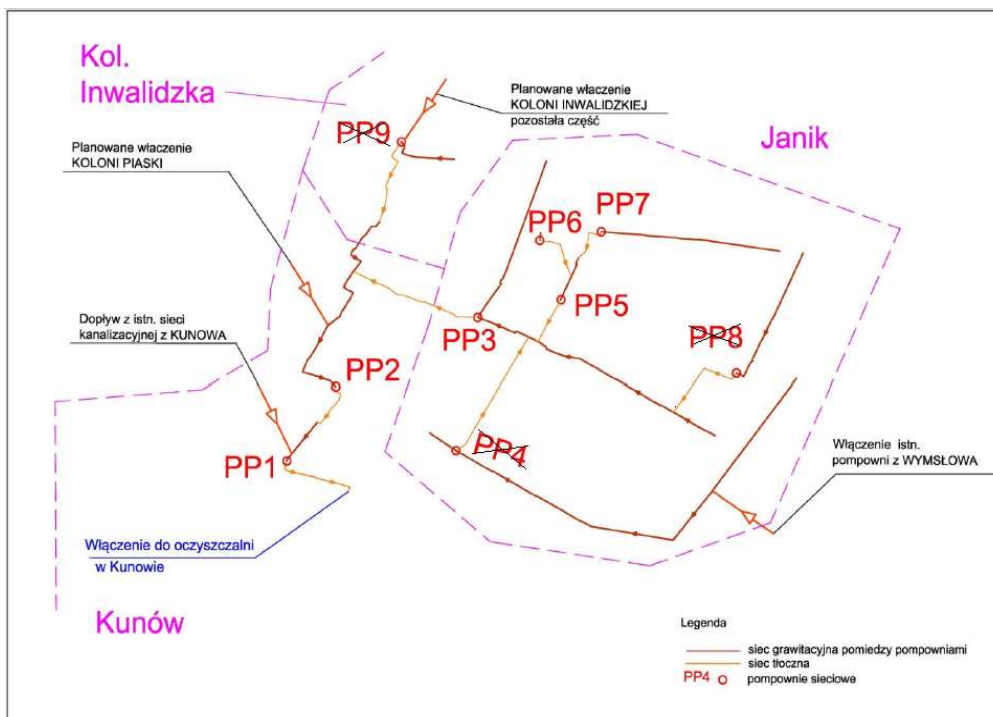
Rysunek 36. Zakres projektowanej sieci kanalizacyjnej
