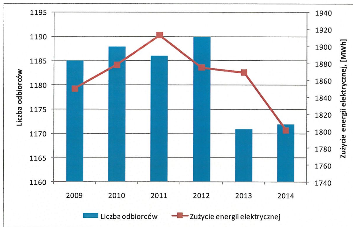
RYSUNEK 5. ZUŻYCIENIE ENERGII I LICZBA ODBIORCÓW W OKRESIE 2009 – 2014 28
