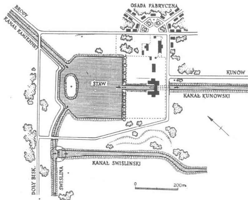
RYSUNEK 16. WALCOWNIA W NIETULISKU DUŻYM – UKŁAD PRZESTRZENNY 7
